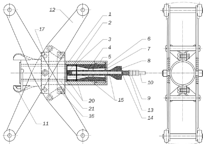
Chariot de centrage ajustable.
